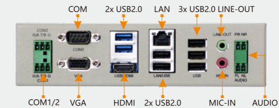
前面板接口
