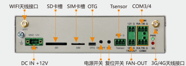
后面板接口
