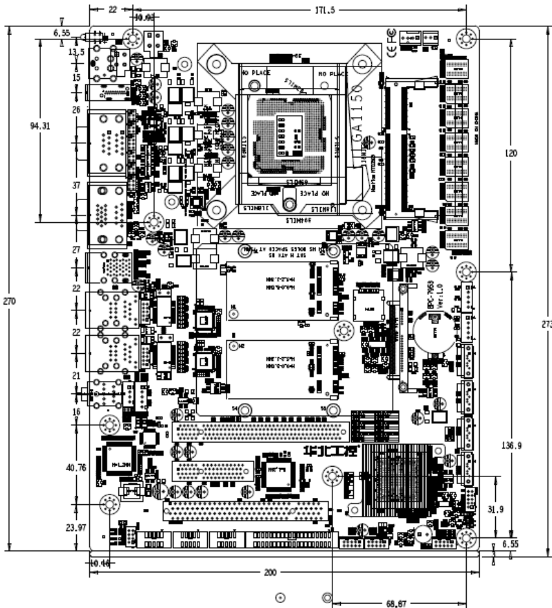
BPC-7953 接口位置和尺寸图
