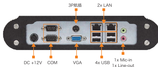
BIS-6650D接口
