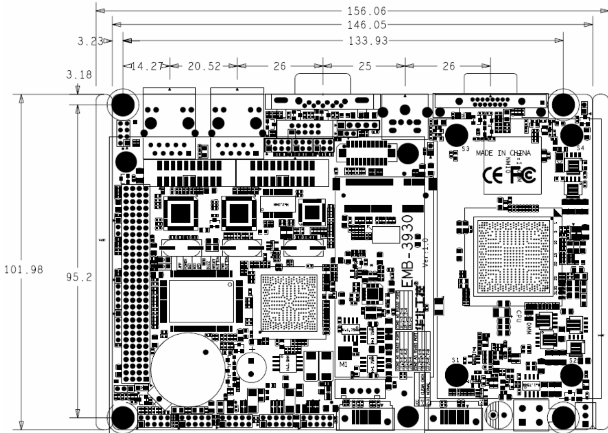
EMB-3930 尺寸和接口位置图
